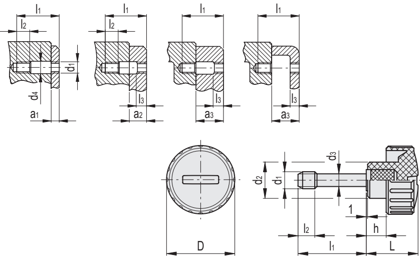
Montagearten
