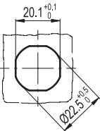
Montagebohrung
