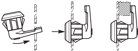
Montagebohrung
