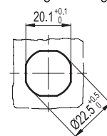
Montagebohrung
