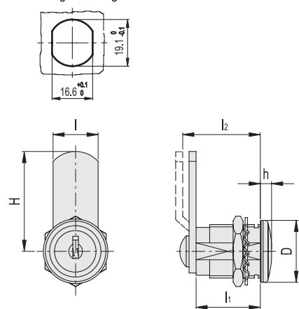
Montagebohrung
