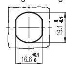
Montagebohrung
