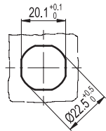
Montagebohrung
