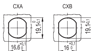
Montagebohrungen
