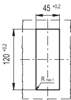
Montageschablone (Bohrung vor der Montage entgraten)
