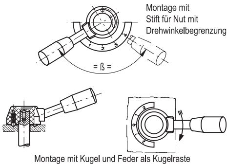
Einbaubeispiel
