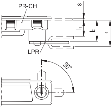
Montage von Griffmulden PR-CH
