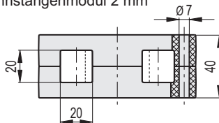
Abmessungen Zahnstange
