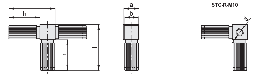
Die Zeichnung zeigt die zusammengebauten Steckverbinder. Die beiden Thermoplast Teile können, abhängig von Größe und / oder Ausführung, unterschiedlich aussehen.
