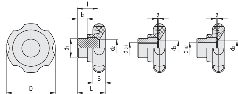
VL.640-FP VL.640-FP-B
