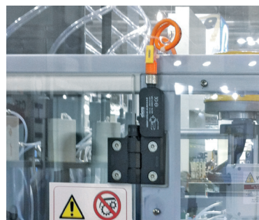
Anwendung des CFSQ Scharniers mit integriertem Sicherheitsschalter.
