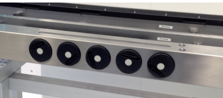
Anwendungsbeispiel der VDS+IRS Scheibenhandräder mit Sicherheits-Umleggriffen
